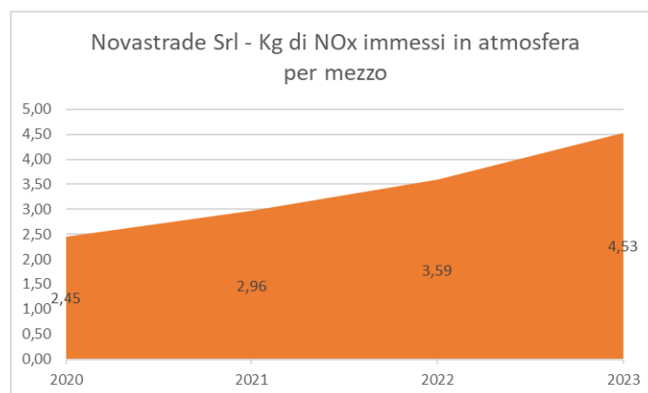
Fig. 21 – NOx medi per mezzo immessi in atmosfera.
